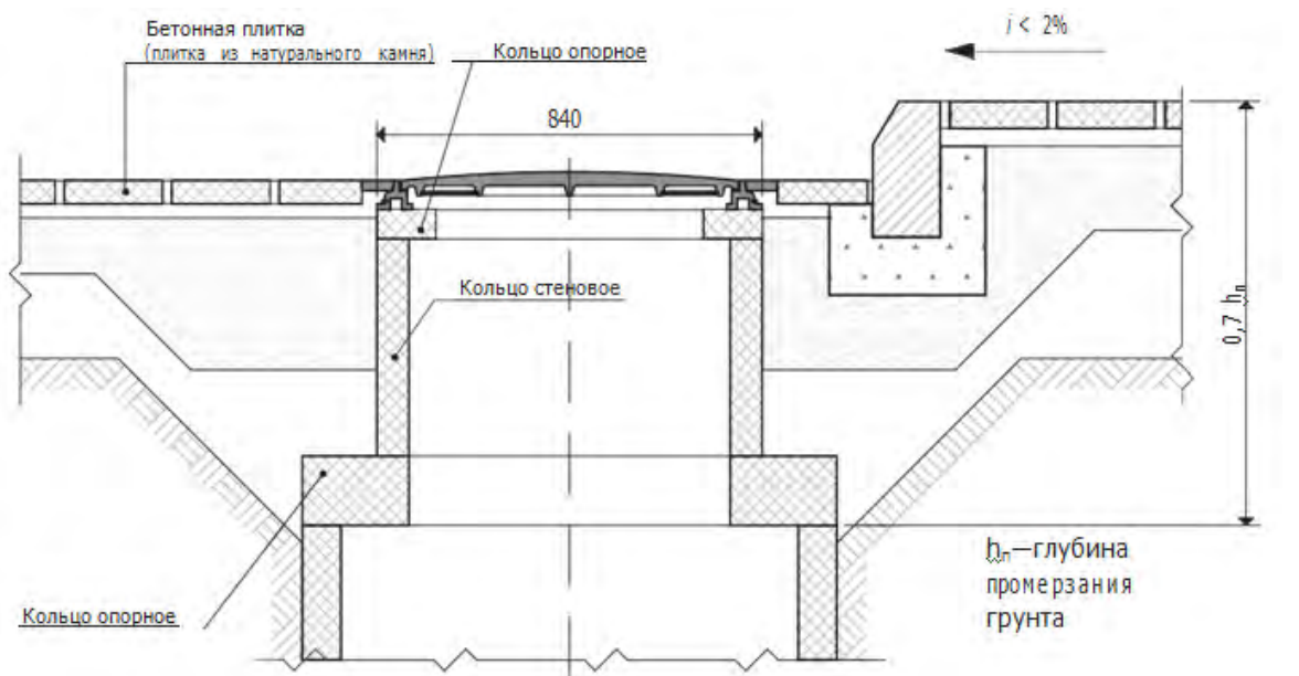
Сечение А-А
